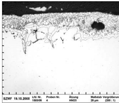
Figuur 6.b - Dompelbad thermisch verzinkt. vergroting 200:1 (bron:Geberit)
